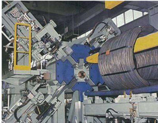
W/ROD 결속
